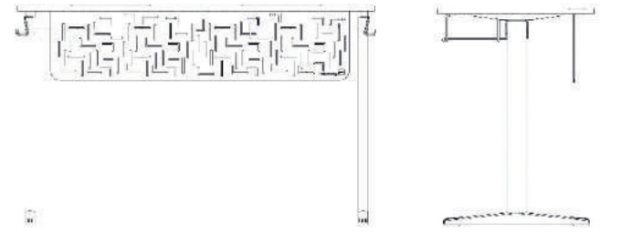
ÜRÜN KODU: 1012113-C Malavi Öğrenci Sırası / Malavi Student Desk Tabla/Desk Top: Kontra Lam 18 mm Ölçü/Size: L:120 W:50 H:64/70/76 Ön Panel/Front Panel: Metal Ön Panel
