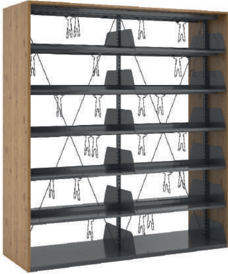
ÜRÜN KODU: 107214 Çiftli Çift Yüzlü Metal Rafı Ahşap Kitaplık Ölçü/Size: L:182 W:62 H:205
