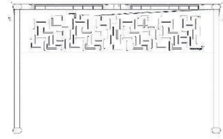
ÜRÜN KODU: 1012212-C Baykal Öğrenci Sırası / Baykal Student Desk Tabla/Desk Top: Kompakt Laminat 12 mm Ölçü/Size: L:120 W:50 H:64/70/76 Ön Panel/Front Panel: Metal Ön Panel
