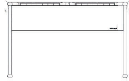
ÜRÜN KODU: 1012212-B Baykal Öğrenci Sırası / Baykal Student Desk Tabla/Desk Top: Kompakt Laminat 12 mm Ölçü/Size: L:120 W:50 H:64/70/76 Ön Panel/Front Panel: MYL Ön Panel
