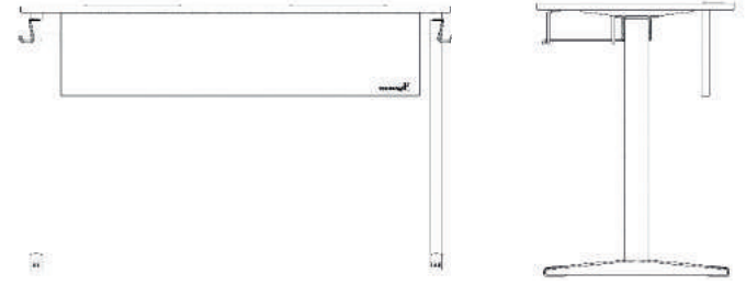
ÜRÜN KODU: 1012113-B Malavi Öğrenci Sırası / Malavi Student Desk Tabla/Desk Top: Kontra Lam 18 mm Ölçü/Size: L:120 W:50 H:64/70/76 Ön Panel/Front Panel: MYL Ön Panel
