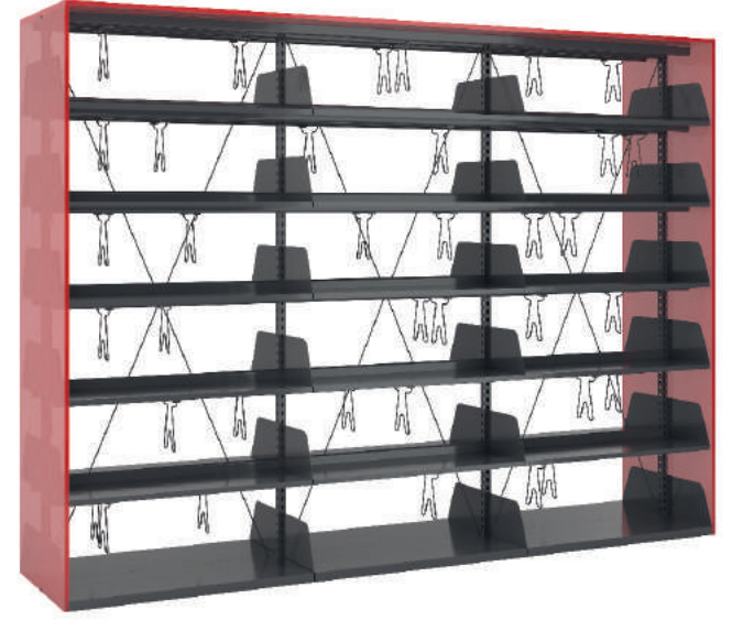
ÜRÜN KODU: 107226 Çiftli Tek Yüzlü Metal Rafı Pleksi Kitaplık Ölçü/Size: L:273 W:62 H:205
